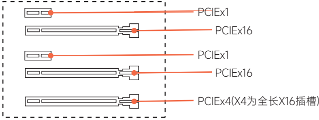
图2-3 PCI扩展插槽
