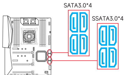
图2 -10 SATA接口
